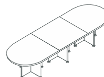
art. KP3T1Q2SL cm. 345 x 115 x 73,3 h.
